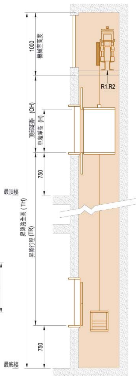
升降路斷面圖
