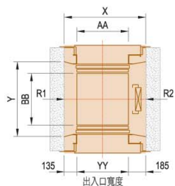
升降路平面圖(T型)
