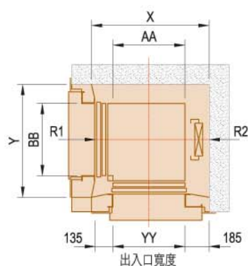
升降路平面圖(P型)
