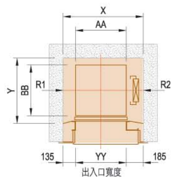
升降路平面圖(S型)
