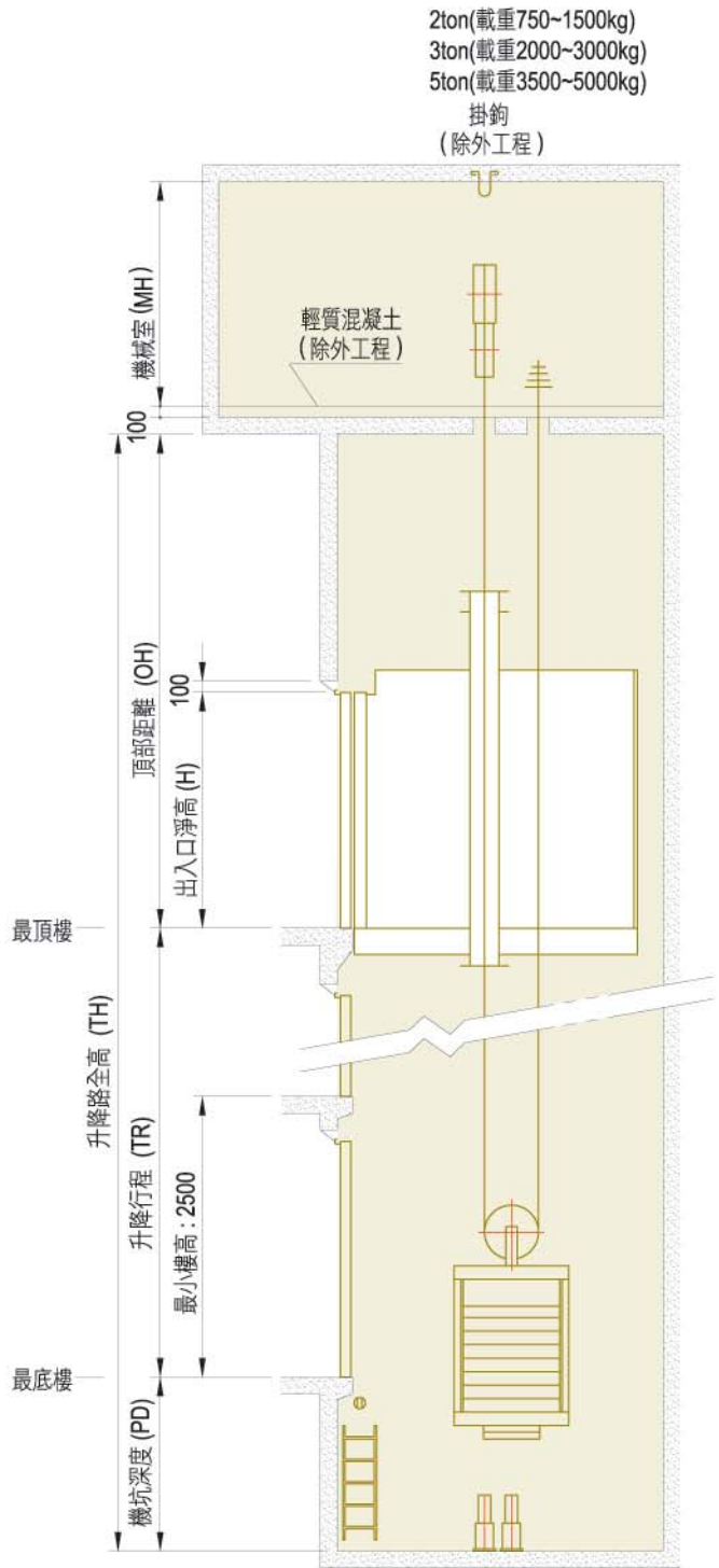
升降路斷面圖
