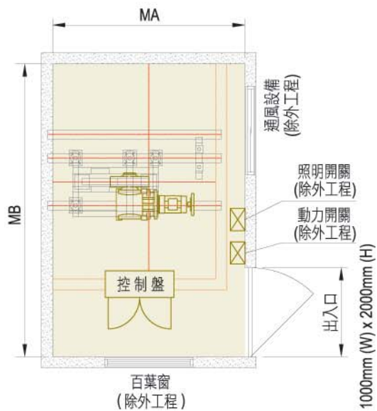
機械室平面圖
