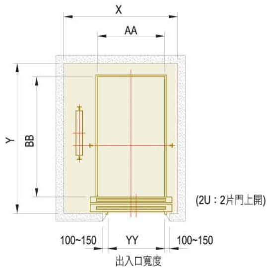
升降路平面圖
