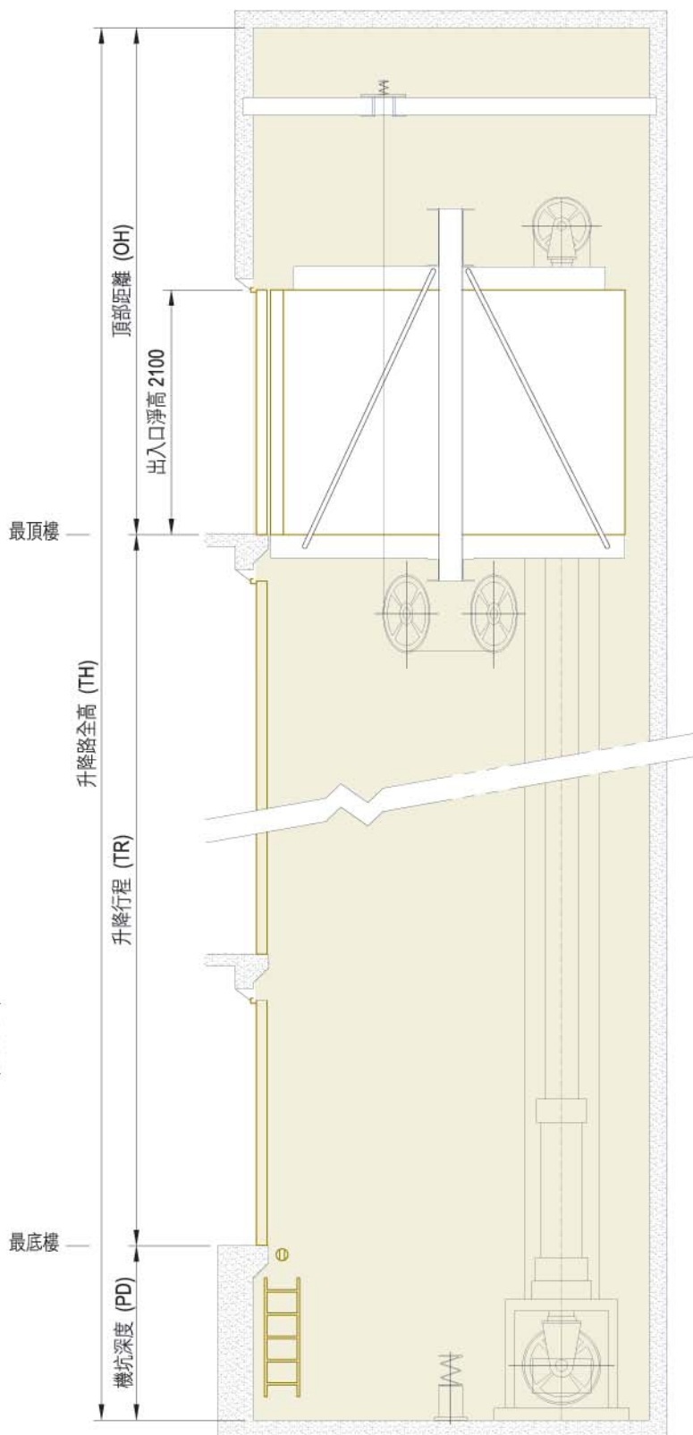
升降路斷面圖
