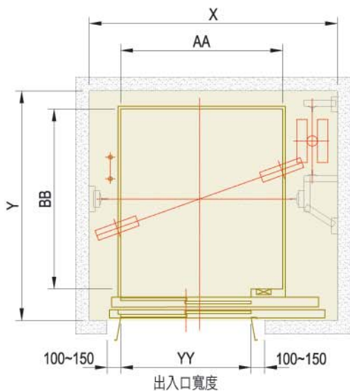
升降路平面圖
